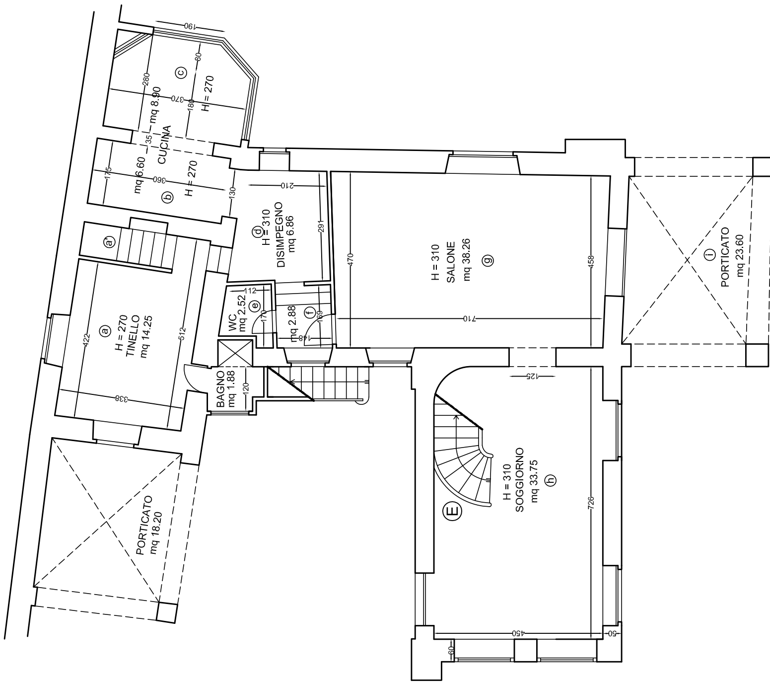
PIANO TERRA – SITUAZIONE ATTUALE
