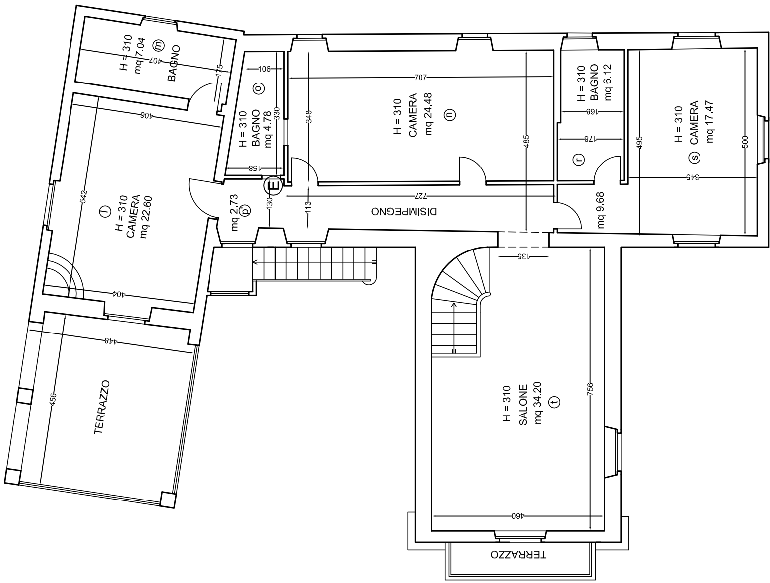
PRIMO PIANO – SITUAZIONE ATTUALE
